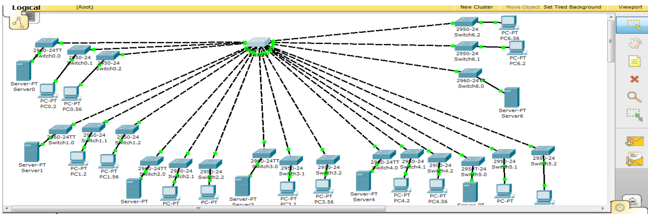
Рисунок 2.1 – Модель мережі
