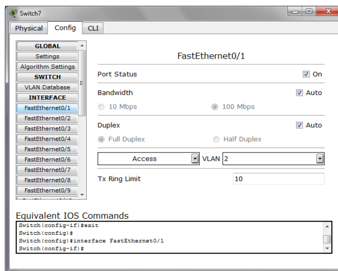
Рисунок 3.3 – Скриншот налаштування портів для підмереж
