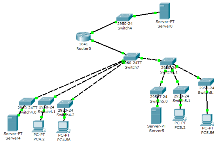
Рисунок 3.1 – Модель мережі
