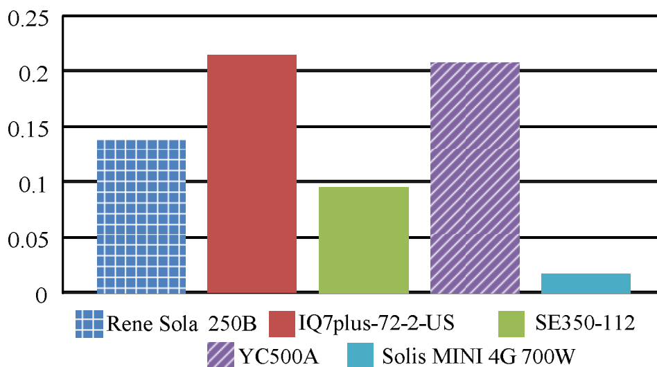
Рис. 6. Питома об'ємна вартість P &lt; 1 кВт
