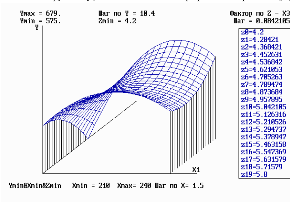
Рис. Маргінальна поверхня відгуку \hat{y}_1 для факторів X_1 і X_3 при X_2 = 120
