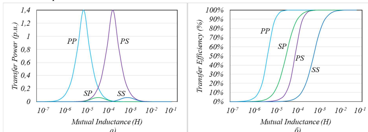
Рис. 2. Порівняння залежностей від взаємоіндуктивності для базових топологій: а – передана потужність; б – ефективність
