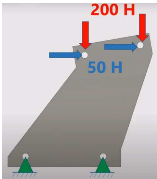
Рис. 1. Розрахункова модель
