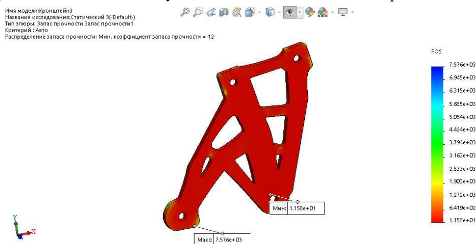
Рис. 5. Еюра запасу міцності
