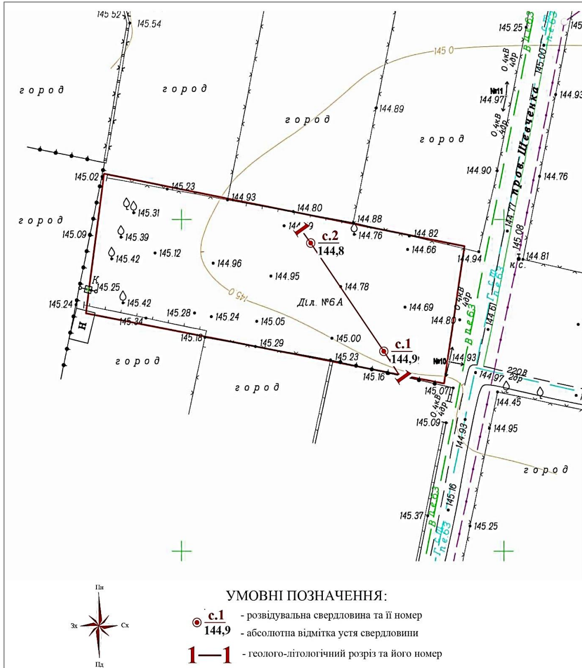
Рис. 2. План розташування свердловин, М 1:500
