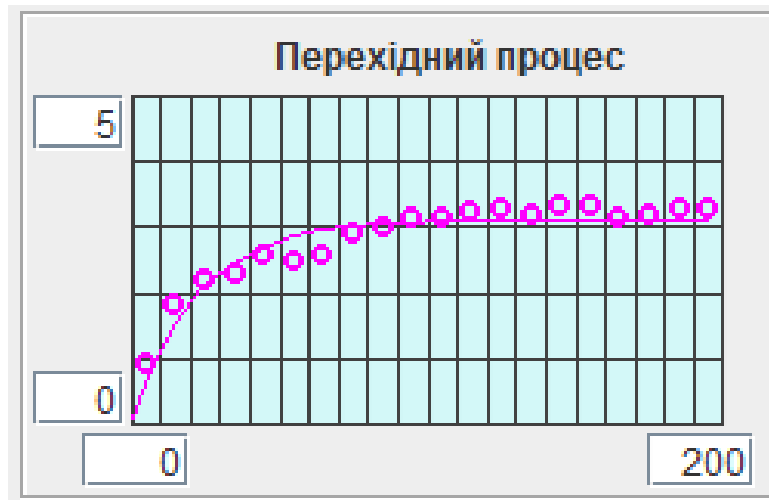
Рисунок 7.3 – Перехідний процес для СМО M/M/1/\infty
