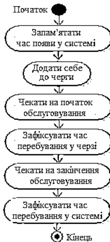
Рисунок 4.1 – Діаграма діяльності абстракції транзакції
