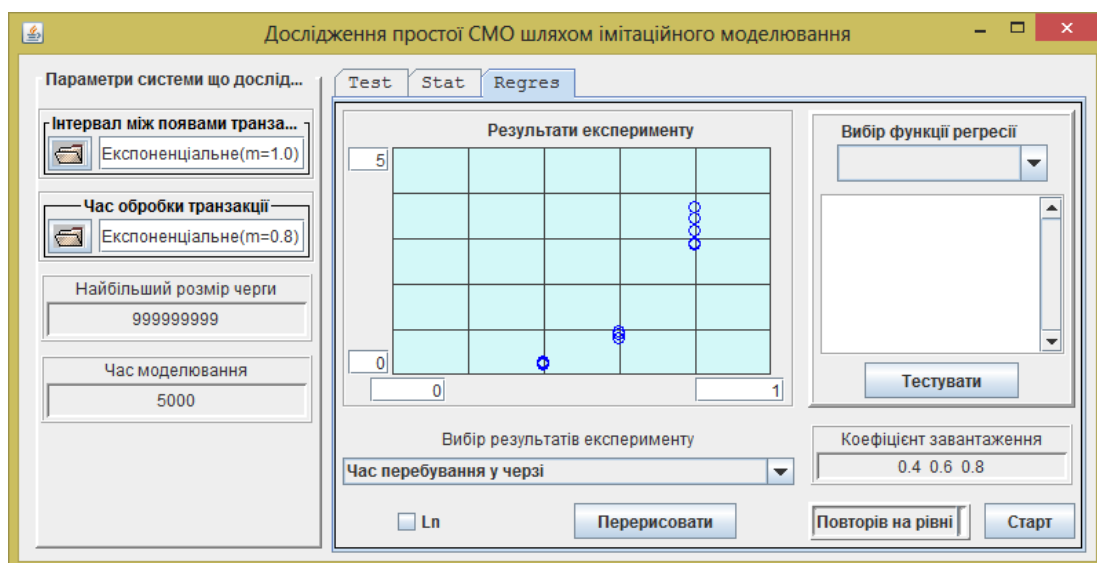
Рисунок 6.6 – Візуальна композиція класу ExperimentUI
