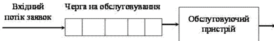
Рисунок 3.2 – Схема найпростішої СМО
