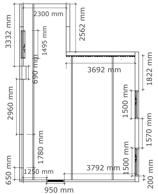
План з розмірами
