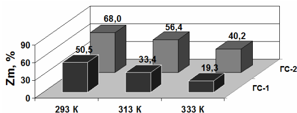
Рис. 4. Зависимость эффекта «последствия» ингибиторов ГС-1 и ГС-2 от температуры раствора 1n HCl на стали Ст3 (экспозиция 2 часа)
