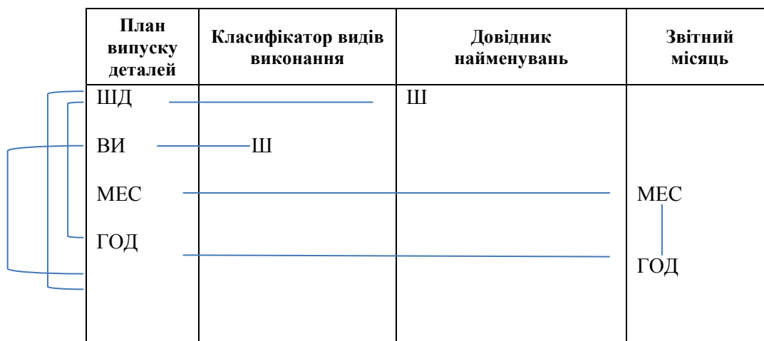
Рис. Графічне відображення зв'язків таблиць у запиті
